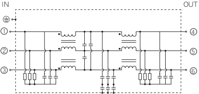
电路图
