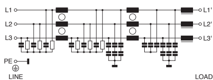
回路図
